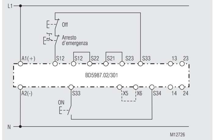
Circuito arresto d'emergenza ad un canale. Questo circuito non ha alcuna ridondanza nel circuito fincorsa arresto d'emergenza. Adatto fino a SIL2, Performance Level d, categoria 3
