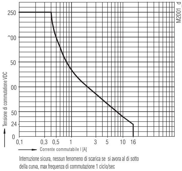
Curva arco limite su carico resistivo
