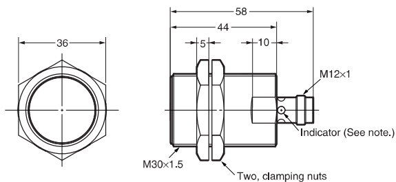
E2A-M30KS15-M1-□□/E2A-S30KS15-M1-□
